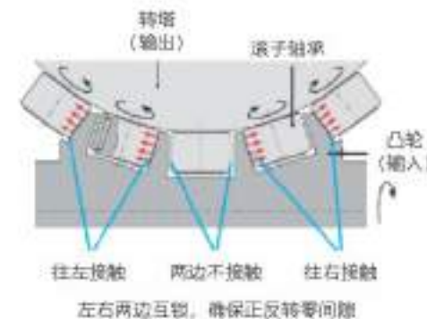
左右两边互锁，确保正反转零间隙
