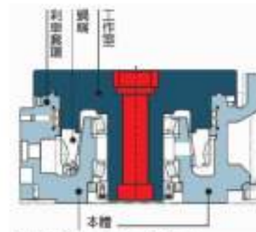
油压全覆周环抱刹車
